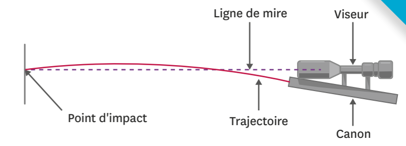
Doc. 5 Trajectoire de la balle lors du tir.
